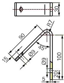
Wandbügel 45°
