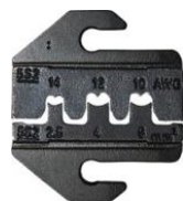
AB MC 4. PRESSBAKKE FOR SOLCELLEKONTAKT ER 2,5-6MM² TIL AB 3
