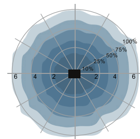
Tunnistusalue seinään asennettaessa (yksikkö: m) Suositeltu asennuskorkeus: 2,5–6 m.
