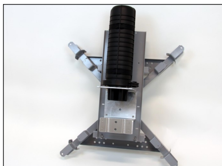
Kveilekryss med skjøteboks, FOSC-OPGW
