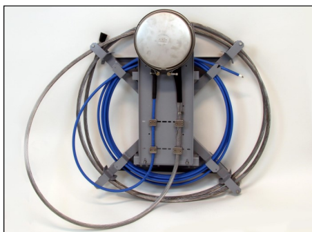
Kveilekryss med Tykoflex skjøteboks, OPGW
