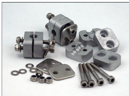
402915-xx - Kabelfeste, OPGW, xx mm, 4 pkn, Alu*
