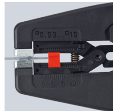
klembakker av stål forhindrer rutsjing av lederen
