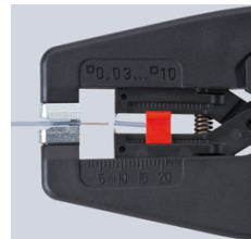
presis avisolering fra 0,03 til 10 mm 2 uten etterjustering
