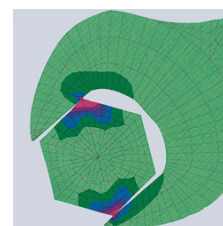
vanlig skrutrekker: kantpressing fører til skade
