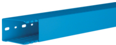
SLISSET KANAL,73X49 H.FRI BLÅ
