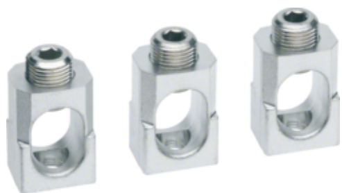
KLEMMER CU 185MM2 3-POL h630 MAX 400
