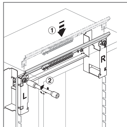
Montering av PE-skinne
