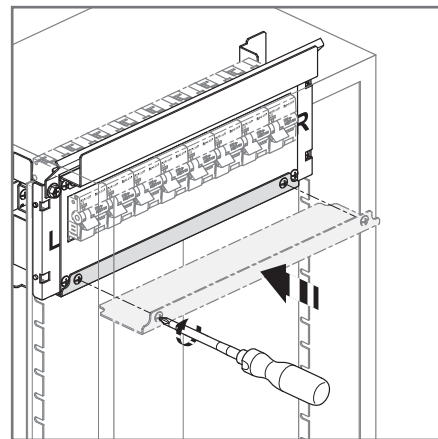
Montering av nedre deksel
