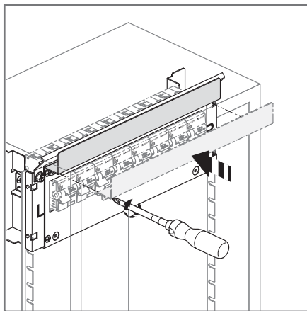
Montering av deksel over PE-skinne
