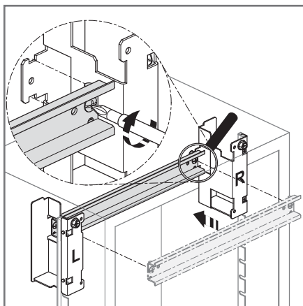
Montering av DIN-skinne
