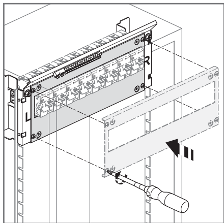
Montering av frontpanel
