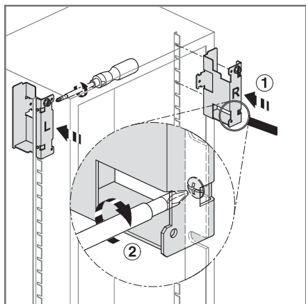
Montering av sidebrakett
