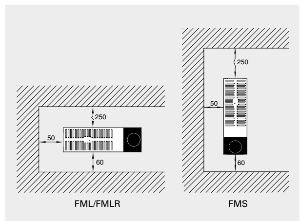
Fig. 1: Minsteavstand ved fast montering.
