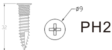
GP 37 Spesialtilpasset skrue for tre og stålstendere som flukter med stenderfeste slik at gipsplater ikke buler. Tilpasset Boks serie R-line 42 - 60 - 72 - 80 - 92 - 120
