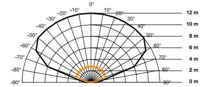
Dekningsområde IS2160 ECO Monteringshøyde 1,8 m Svart – tangential gangretning Oransje – radial gangretning
