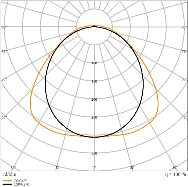
DP 600 P 13W ML 840 VW IP66
