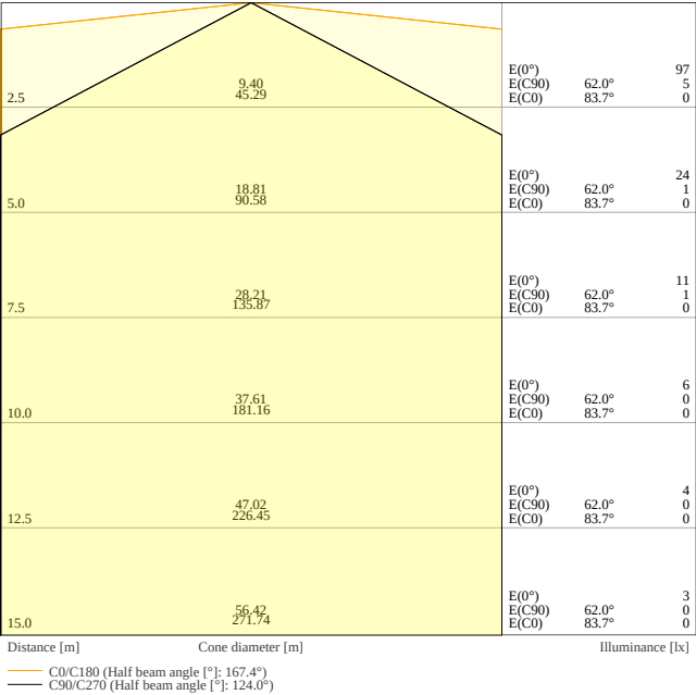
DP 1200 P 26W ML 840 XW IP66
