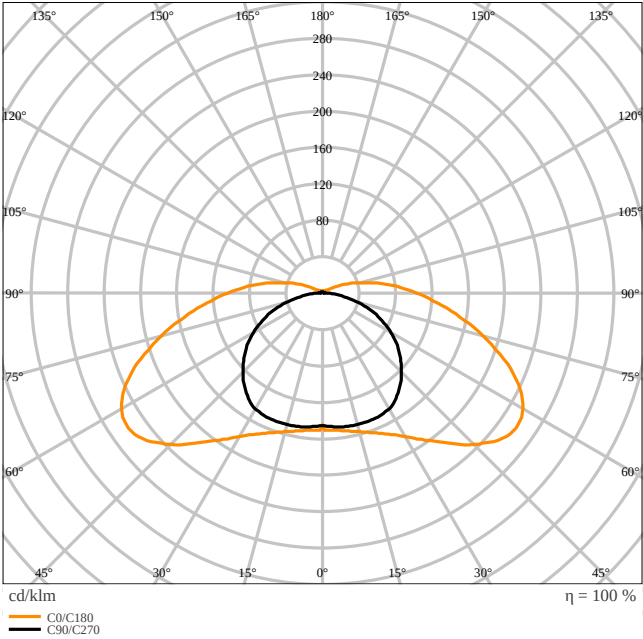
DP 1500 P 36W ML 840 XW IP66
