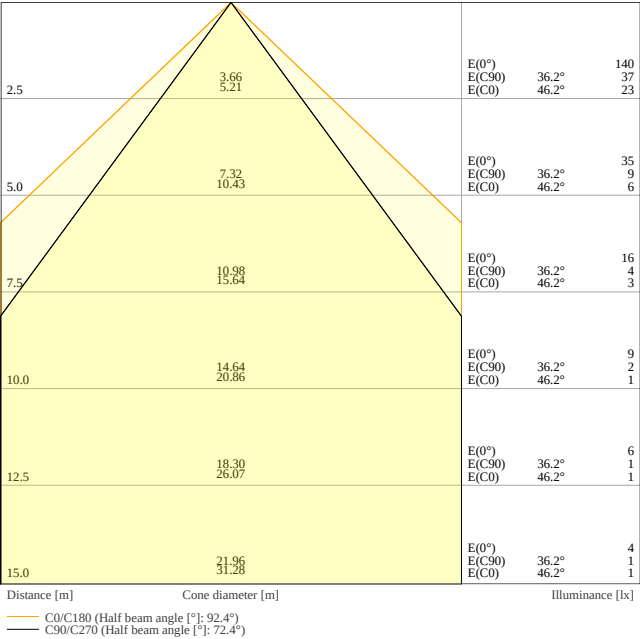
DP 600 P 13W ML 840 VN IP66
