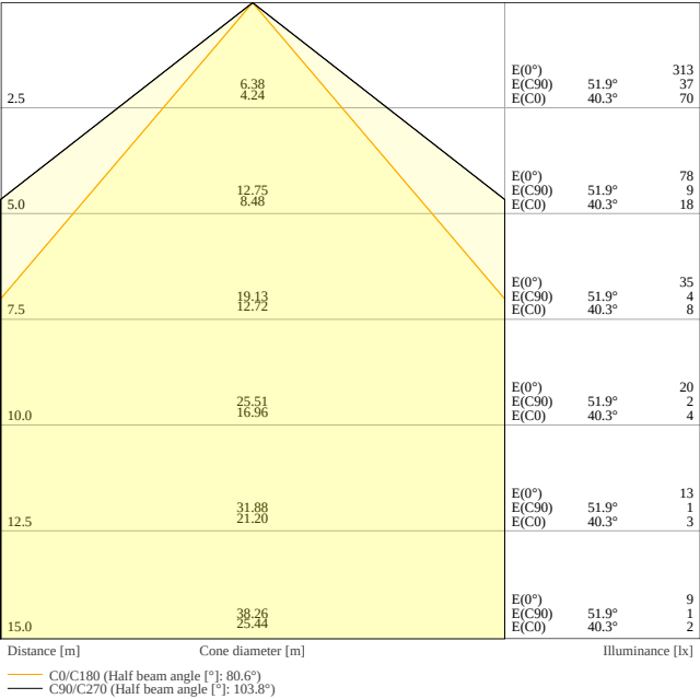
DP 1500 P 36W ML 830 VN IP66
