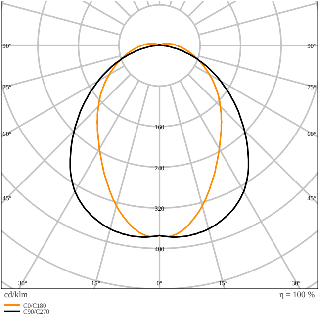
DP 1500 P 36W ML 840 VN IP66
