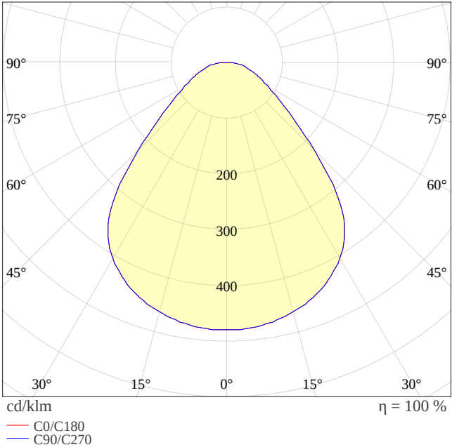
PL CMFT 1200 DA P 24W 830 U19 3840lm
