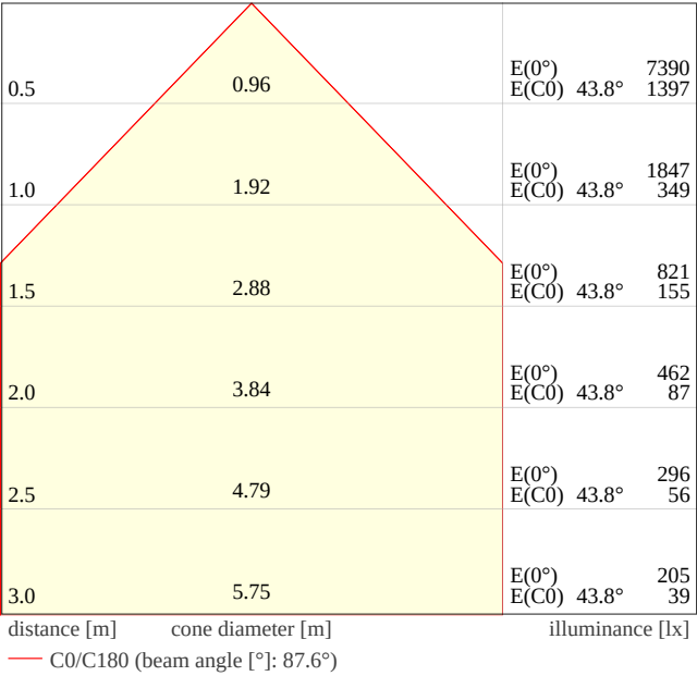
PL CMFT 1200 DA P 24W 830 U19 3840lm
