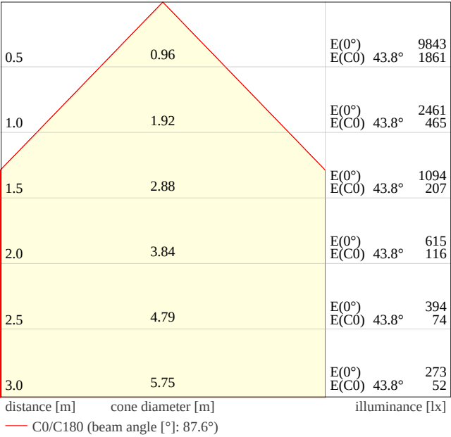
PL CMFT 1200 DA P 33W 830 U19 5115lm
