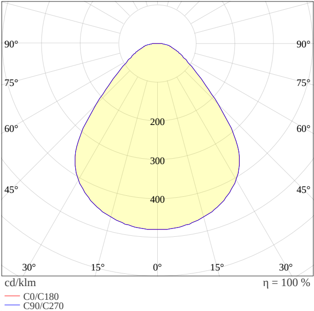
PL CMFT 1200 DA P 33W 940 U19 5115lm
