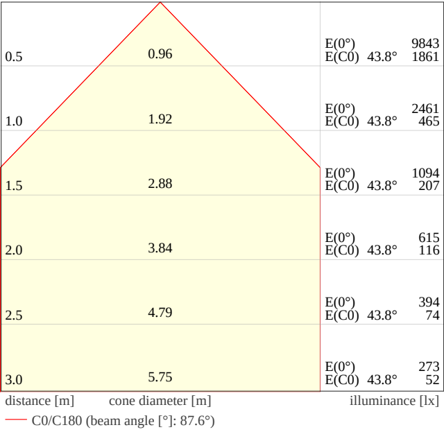
PL CMFT 1200 DA P 33W 940 U19 5115lm
