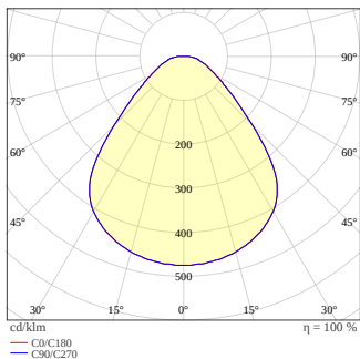
PL CMFT 600 DA P 24W 840 U19 3840lm
