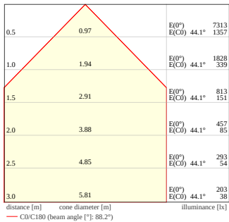
PL CMFT 600 DA P 24W 840 U19 3840lm
