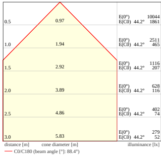
PL CMFT 600 ZB P 33W 830 U19 5280lm
