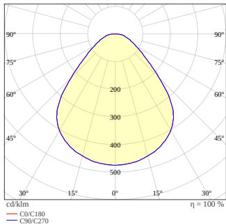
PL CMFT 600 ZB P 33W 830 U19 5280lm
