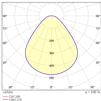
PL CMFT 600 ZB P 33W 940 U19 4950lm
