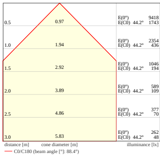
PL CMFT 600 ZB P 33W 940 U19 4950lm
