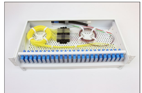
Panel med fiberhaler, SM, skjøtt til kabel
