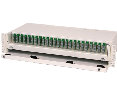
Panel med underliggende 0.5U kabelrenne Totalt 2U
