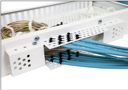
Bakstykke FP70, småkabler
