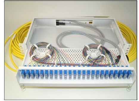
Panel med preterminert kabel, fast kledning
