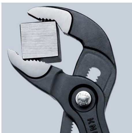
Forskjøvete tenner mot dreieretningen gir en selvklemmende effekt og forhindrer rutsjing på arbeidsstykket
